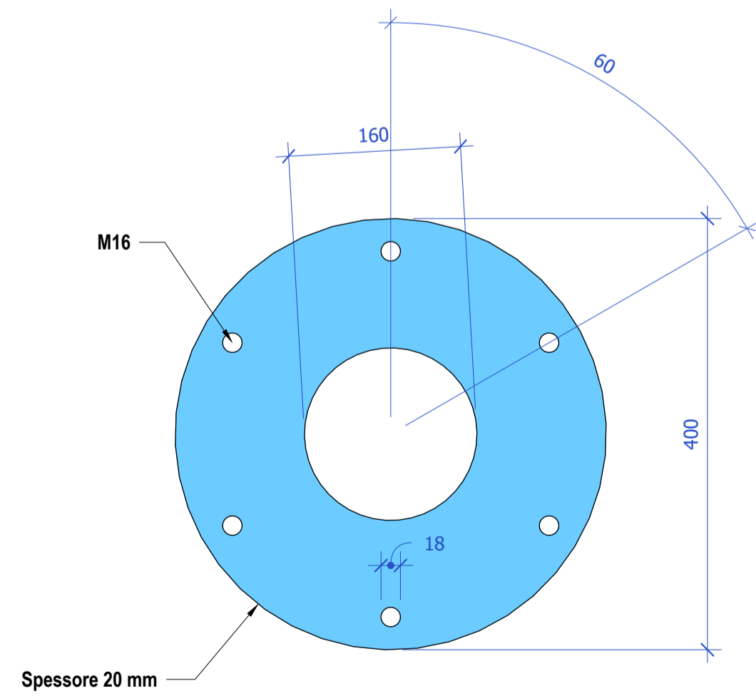
Q LAVORAZIONI SU TUBO X1003 Scale: 1:5
