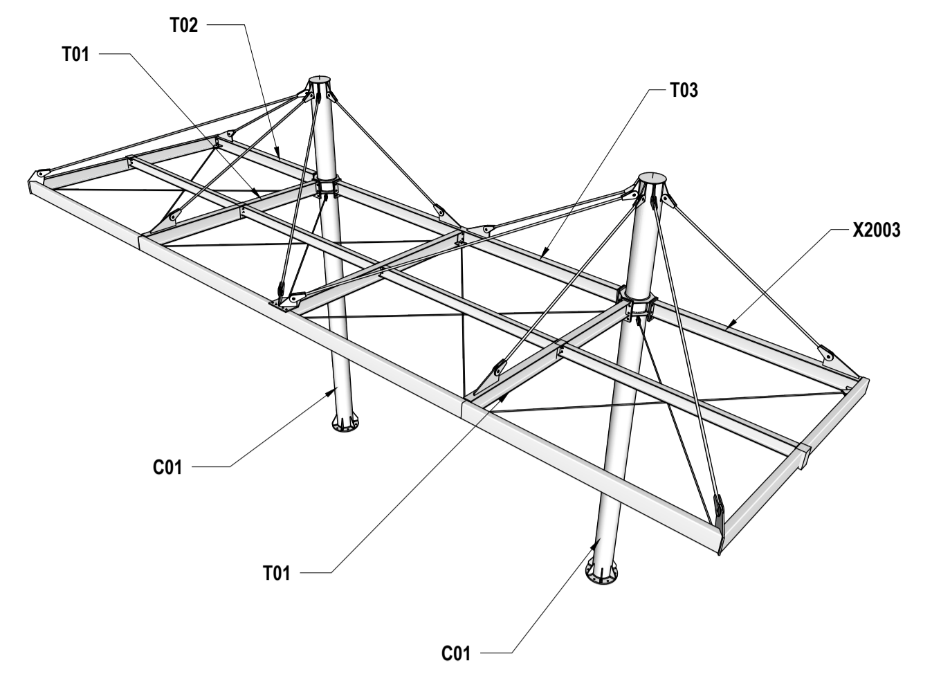
ASSIEME COMPLESSIVO Scale: -
