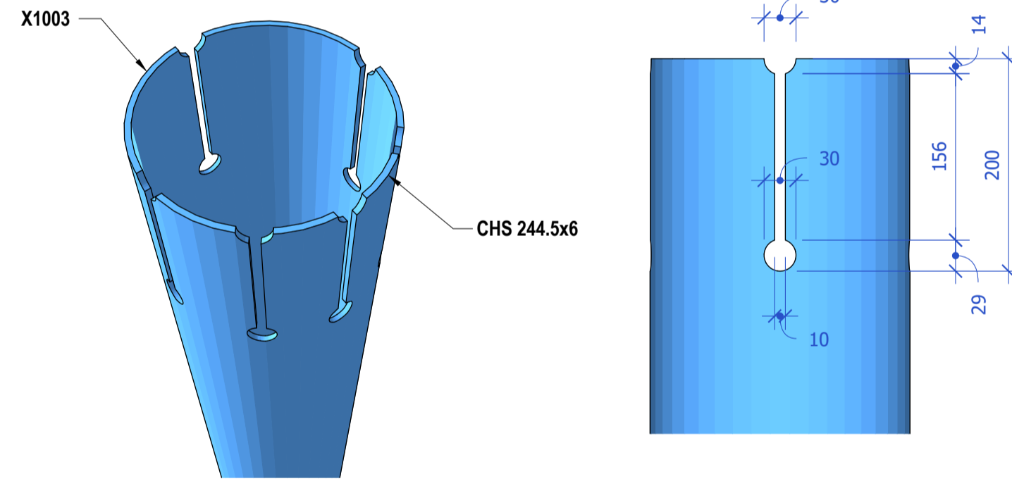
Q LAVORAZIONI SU TUBO X1003 Scale: 1:5
