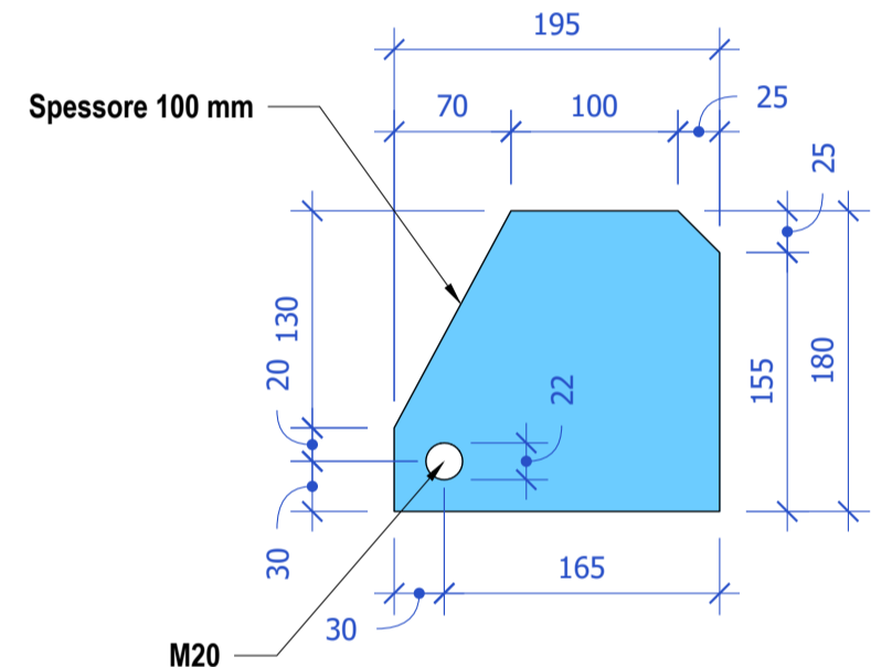
I PARTICOLARE 1009 Scale: 1:5
