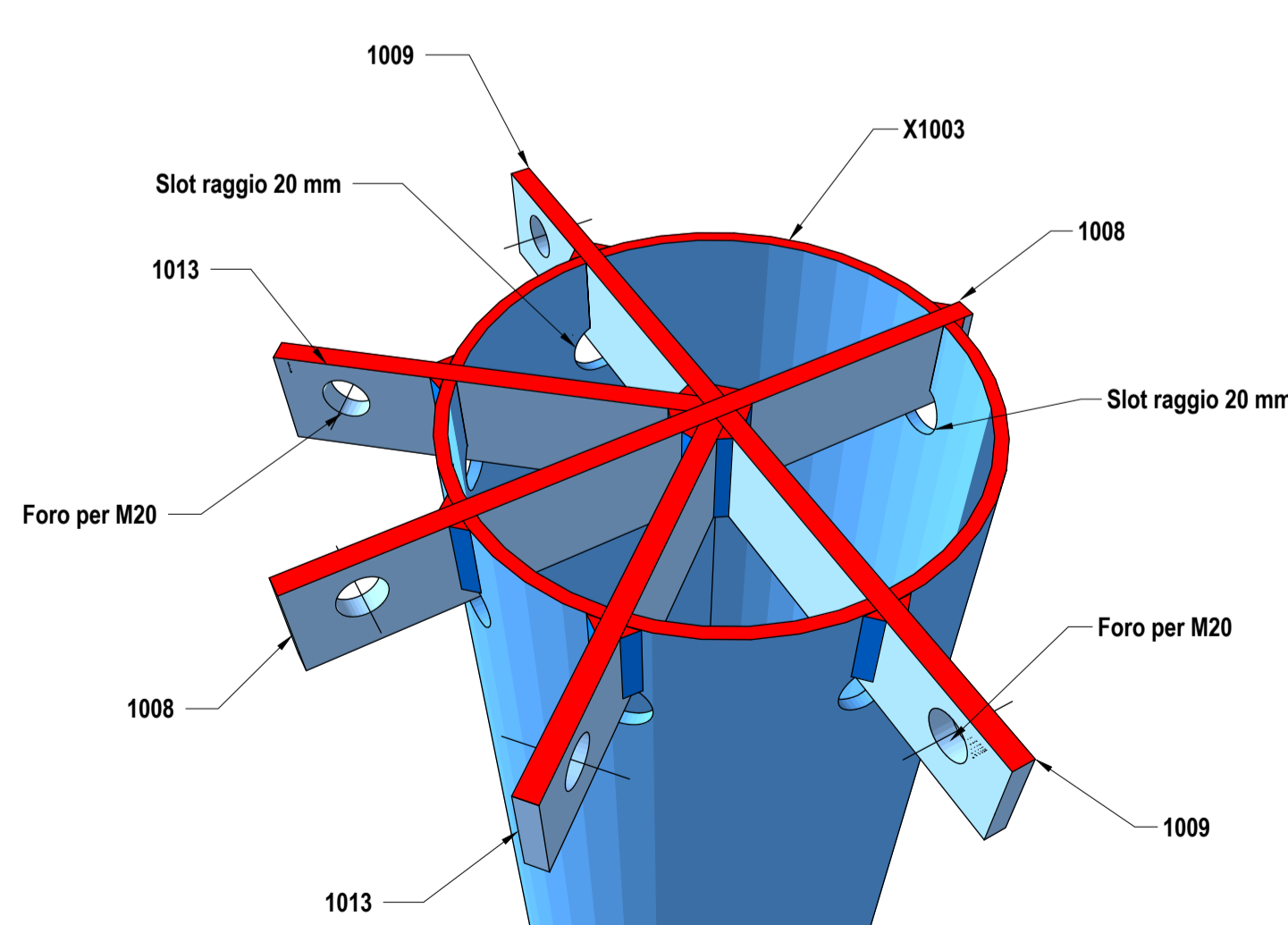
L SEZIONE S3 Scale: -
