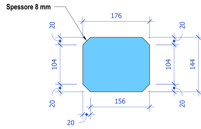
F PARTICOLARE 1004 Scale: 1:5
