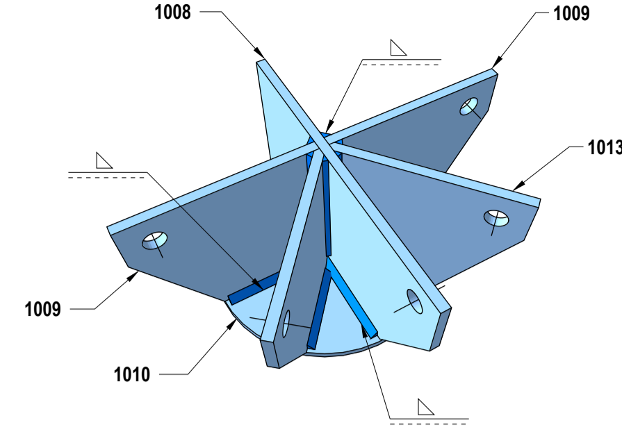
O ASSEMBLAGGIO PIASTRE IN TESTA Scale: 1:5
