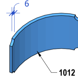
M LAVORAZIONE PARTICOLARE 1012 Scale: 1:5
