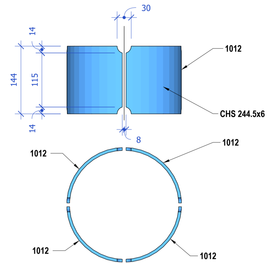
O ASSEMBLAGGIO PIASTRE IN TESTA Scale: 1:5
