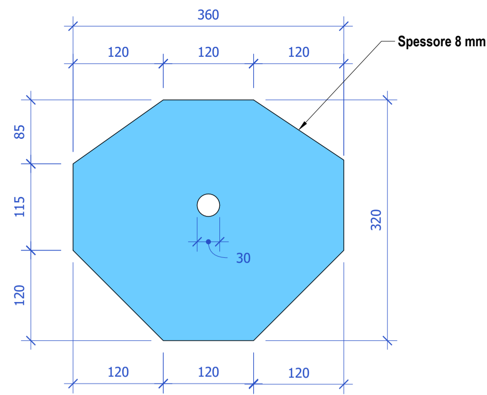
B PARTICOLARE 1003 Scale: 1:5
