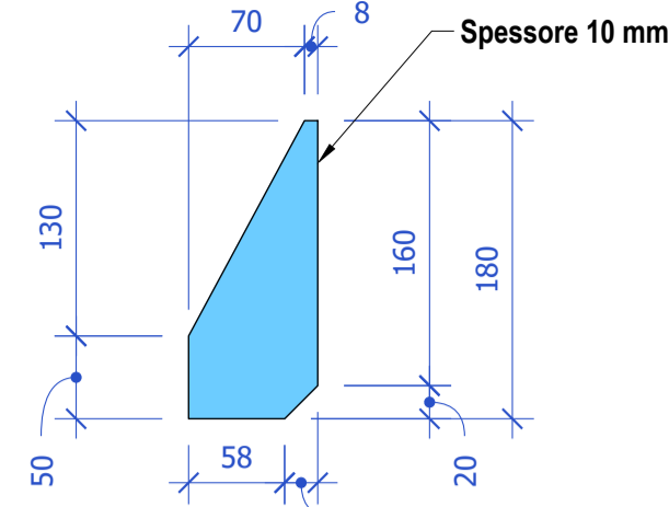
C PARTICOLARE 1002 Scale: 1:5
