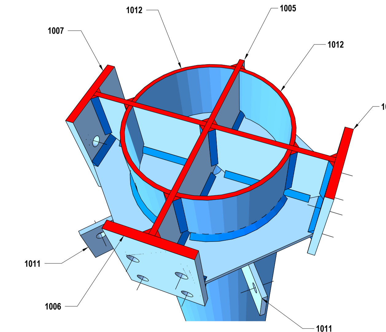
K SEZIONE S2 Scale: -
