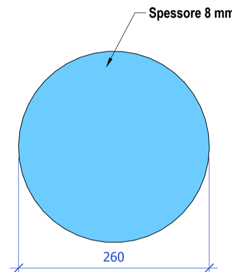
J PARTICOLARE 1003 Scale: 1:5
