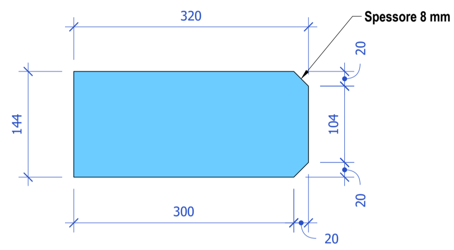
G PARTICOLARE 1005 Scale: 1:5
